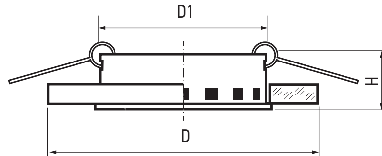
Рис. 1. Светильник PGX53d
